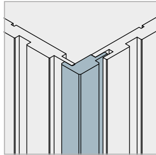
PROFILO ANGOLO QUADRO 276 x 32 x 19 cm
