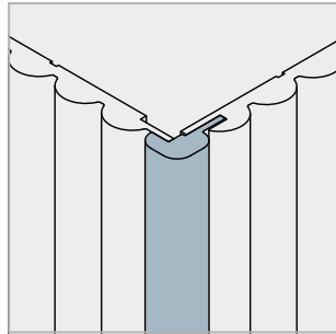
PROFILO ANGOLO TONDO 276 x 29 x 19 cm
